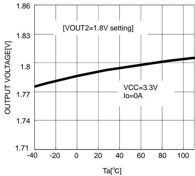
Figure.8 Ta-VOUT2
