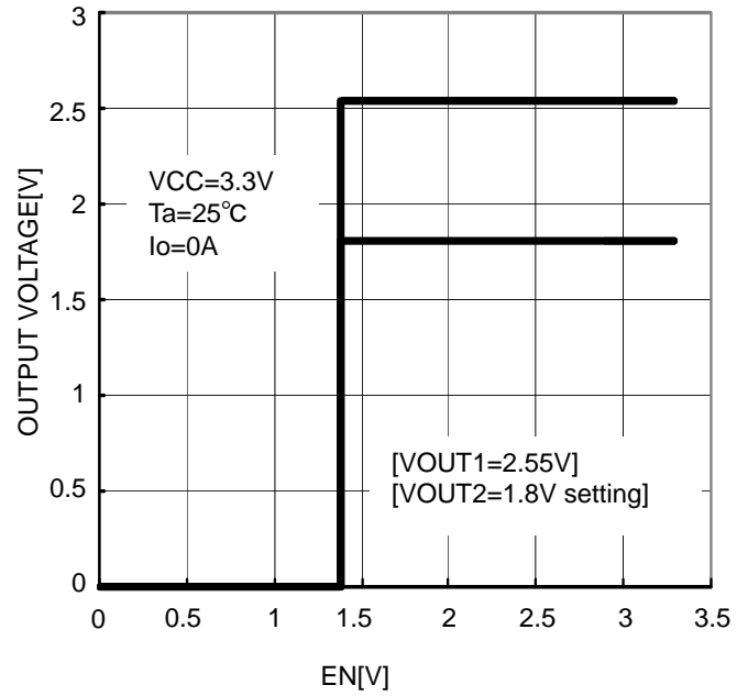
Figure.5 VEN-VOUT
