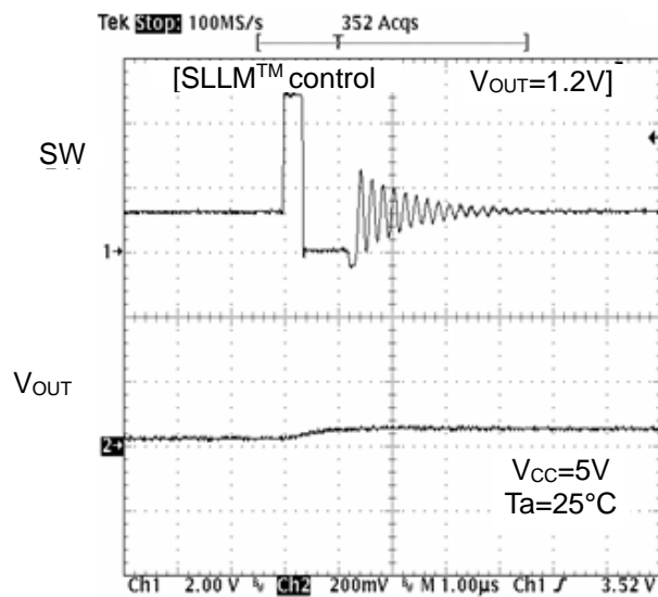
Figure 15. SW Waveform (I O =0mA)
