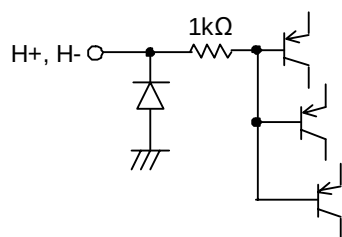
1) Hall input
