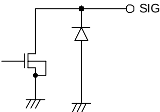
4) SIG output
