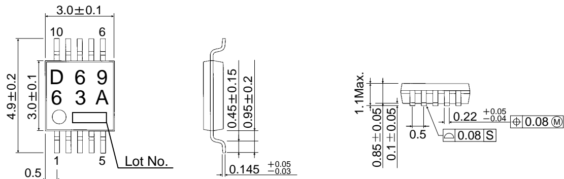
TSSOP-C10J (UNIT:mm)
