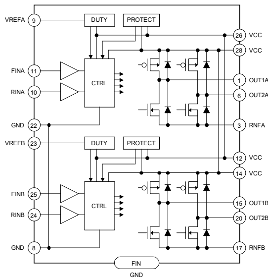
Fig.33 BD6236FM
