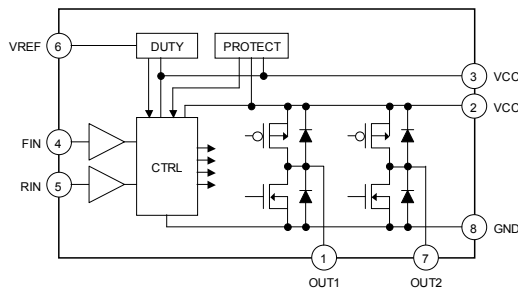
Fig.25 BD6230F / BD6231F
