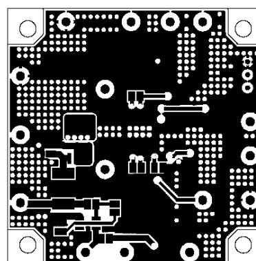
Bottom Layer
