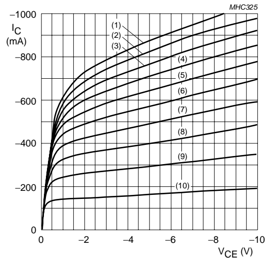
TR2 (PNP)
