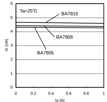
Fig.24 I_o - I_b
