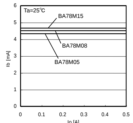
Fig.12 I_o - I_b
