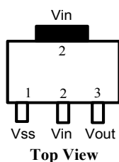
SOT-223 (N)
