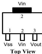
SOT-89 (R)
