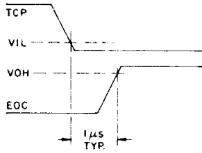
Fig.17 EOC TURN-ON
