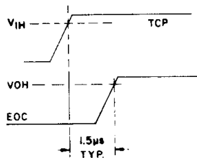
Fig.39 EOC TURN-ON
