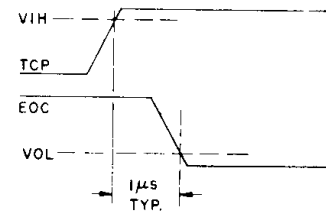
Fig.19 EOC TURN-OFF
