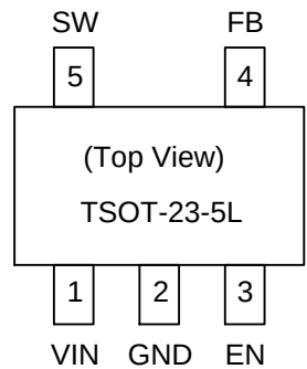
TSOT-23-5L(B Type)
