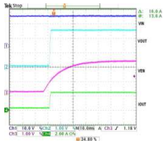
Enable-ON Wave
