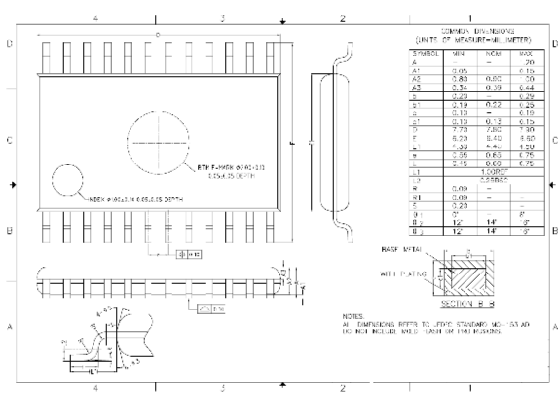
Figure 4 TSSOP24 Package Dimension Parameter
