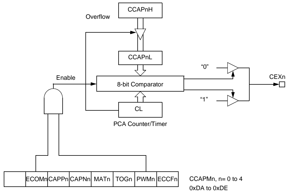
Figure 23. PCA PWM Mode
