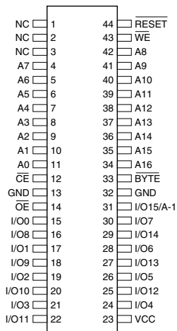
SOIC (SOP)
