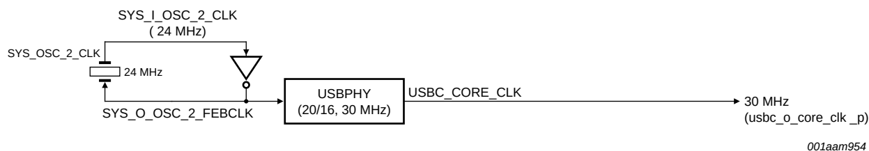
Fig 27. USB clock scheme
