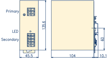
Fig. 2 : Outline dimensions
