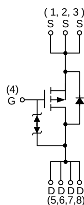
P-Channel MOSFET
