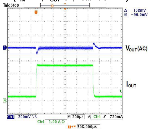
Load Transient (F=60KHz) ( V_{IN}=12V , V_{OUT}=5V , Load=0.3~2.7A)
