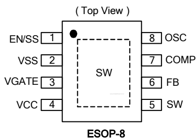
ESOP-8
