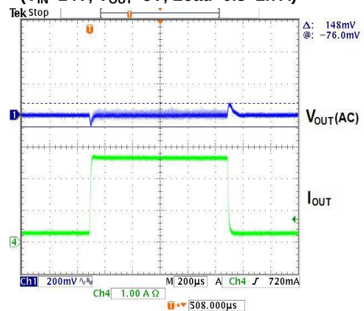
Load Transient (F=60KHz) ( V_{IN}=24V , V_{OUT}=5V , Load=0.3~2.7A)
