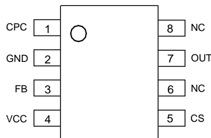
SO-8
