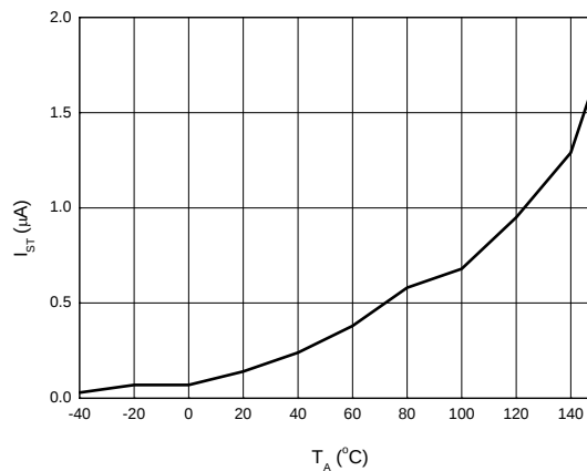
I_{ST} vs. T_A
