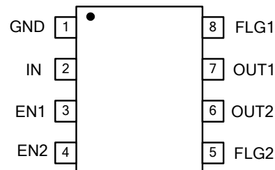
SO-8
