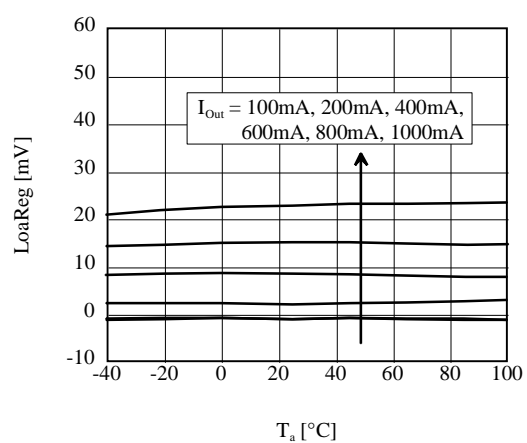
■ \text{LoaReg} vs T_a (AP1155ADU)
