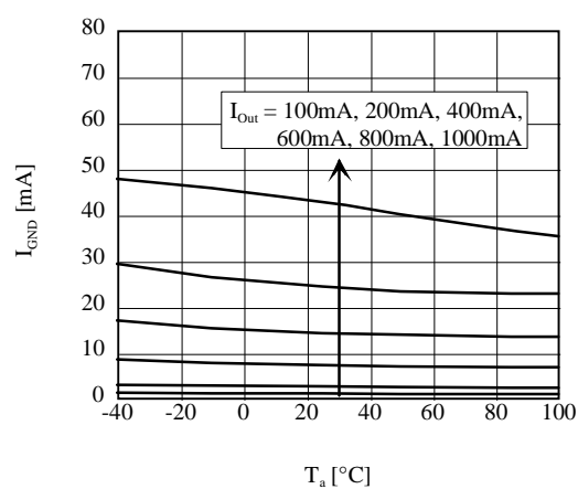
■ I_{\text{GND}} vs T_a (AP1155ADU)
