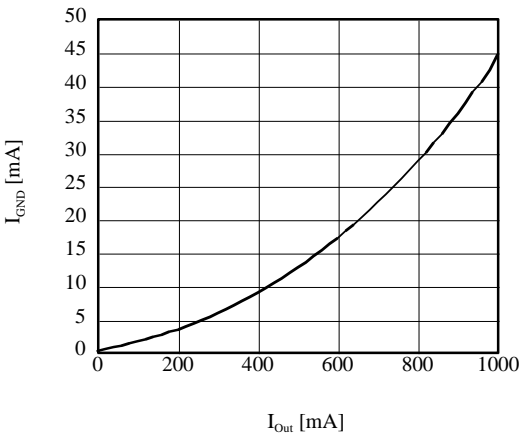
■ I_{\text{GND}} vs I_{\text{Out}} (AP1155ADU)
