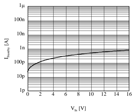
■ I_{\text{Standby}} vs V_{\text{In}} (AP1155ADU)
