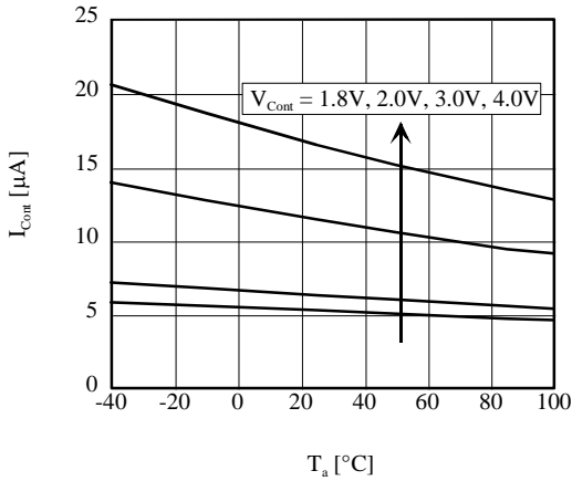
■ I_{\text{Cont}} vs T_a (AP1155ADU)
