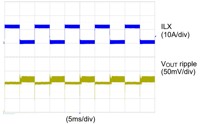
Load Transient 0A to 12A
