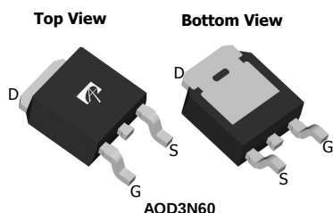
TO252 DPAK
