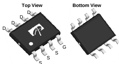
SOIC-8
