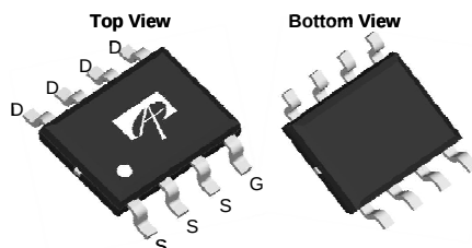
SOIC-8
