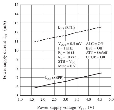
I_{CC7,8} - V_{CC}
