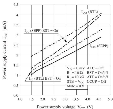
I_{CC} - V_{CC}
