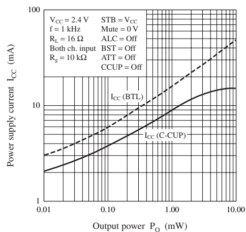
I_{CC} - P_O
