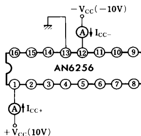
Test Circuit 6 ( I_{CC+} , -I_{CC-} )
