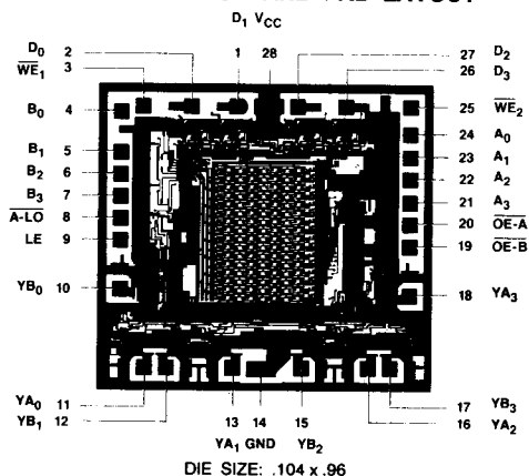
DIE SIZE: .104 x .096
