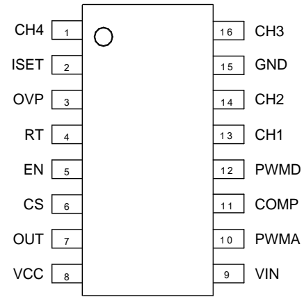
SO-16
