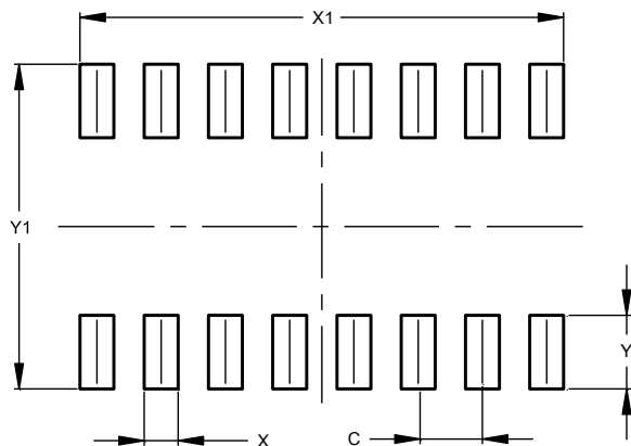
SO-16
