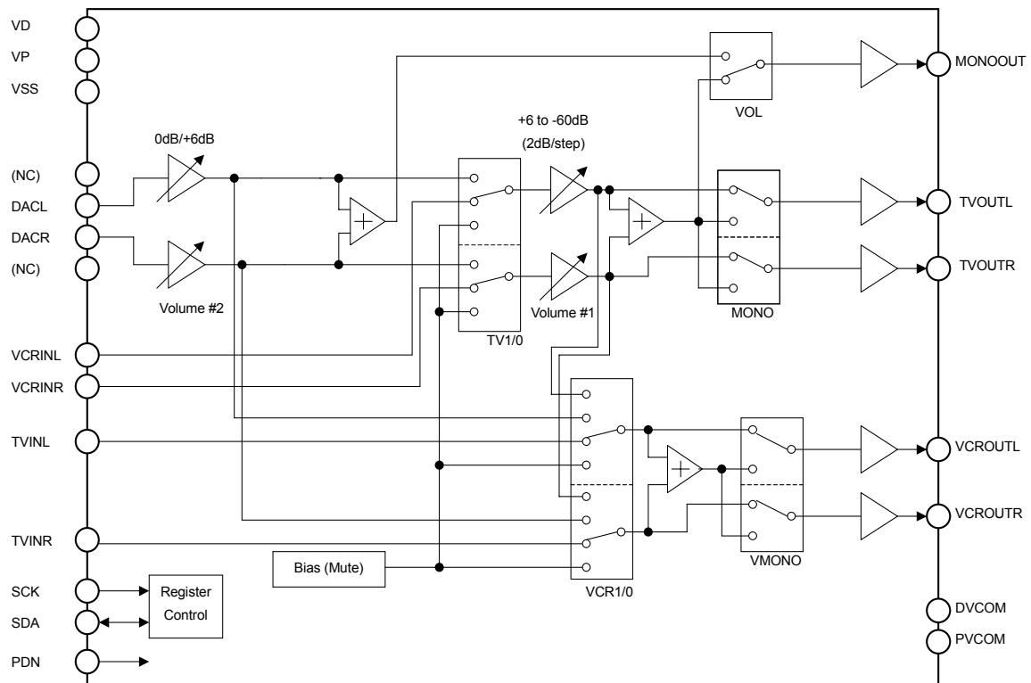
Audio Block(DAPD="1")
