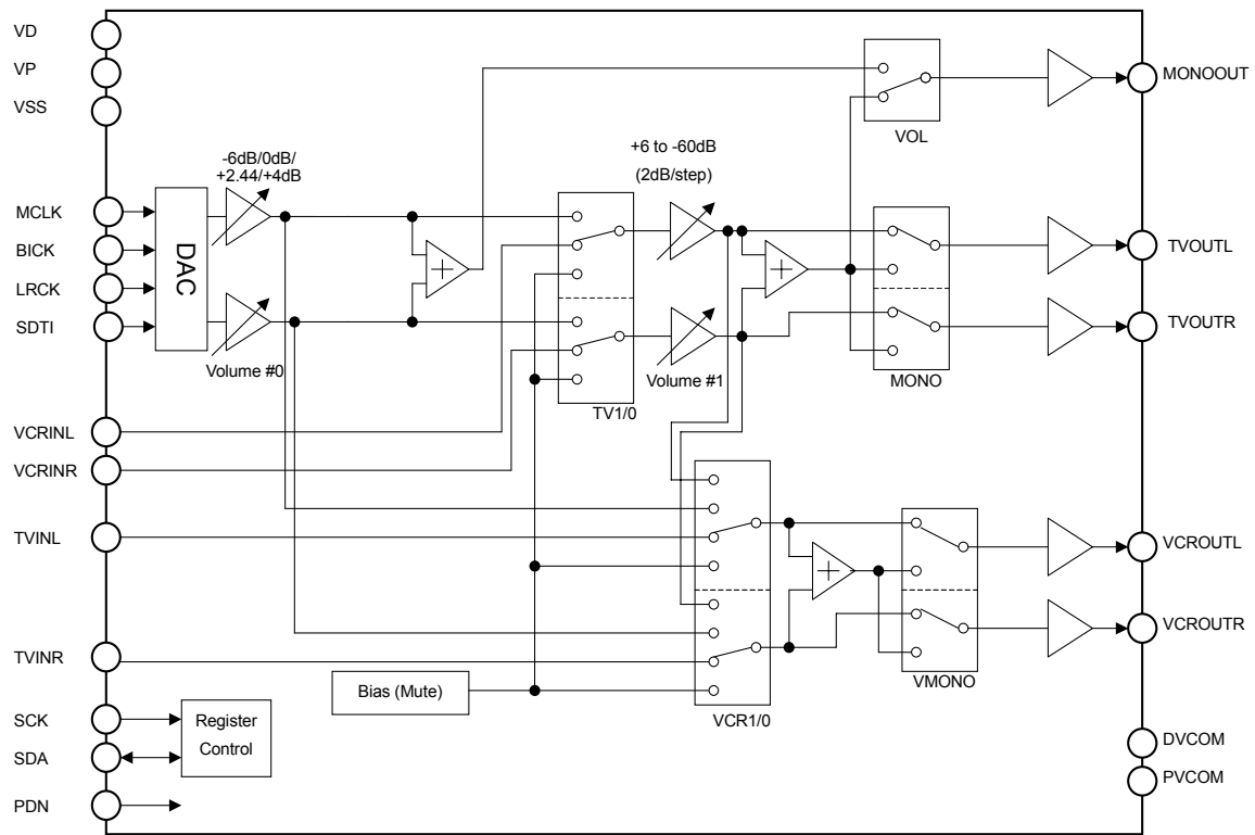
Audio Block(DAPD="0")
