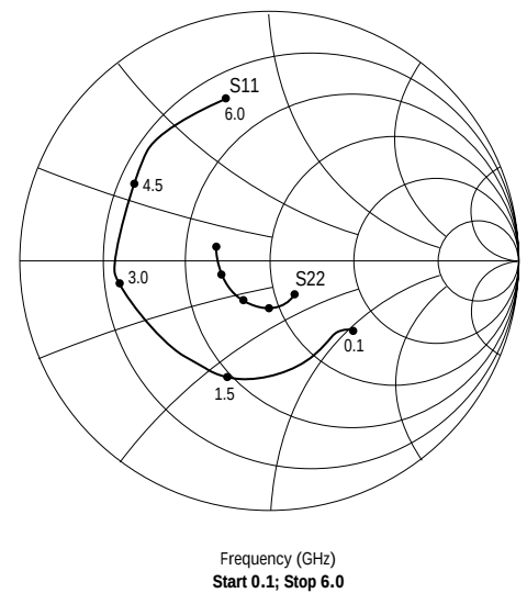
S-Parameters
