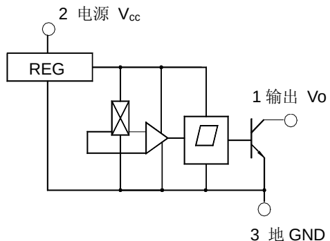
功能方框图
