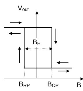
磁电转换特性
