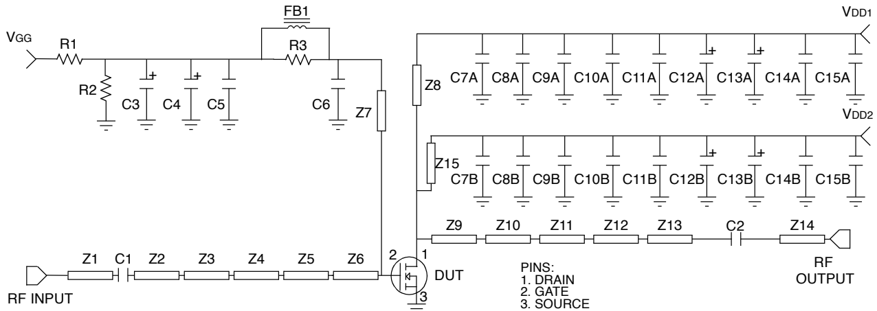
A. Schematic
