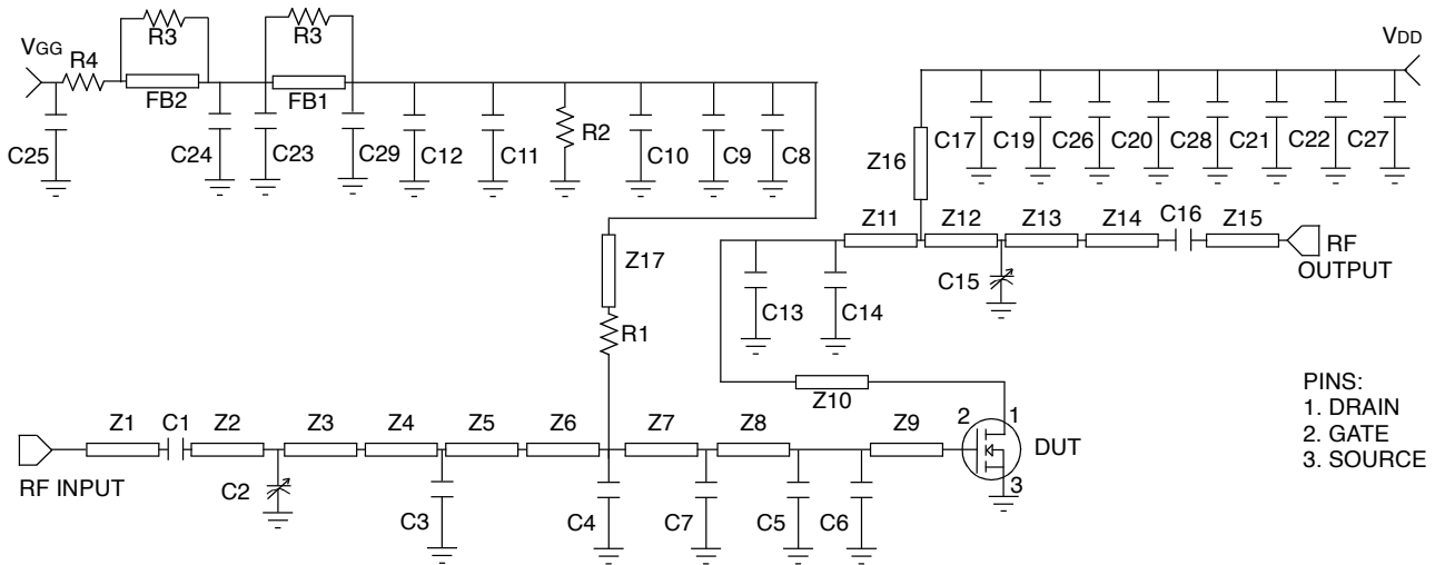
A. Schematic
