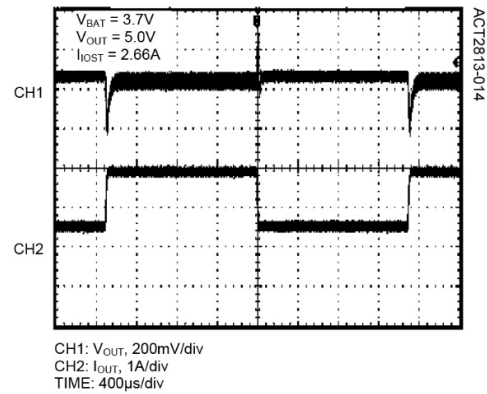
Boost Load Transient (1A-2.4A-1A)
