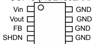
SOP-8 (ACE1502XXFM+)
