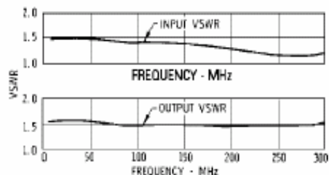
VSWR
