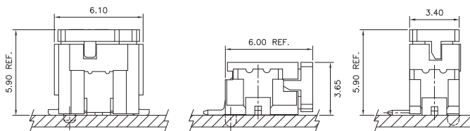
SMT TYPE
