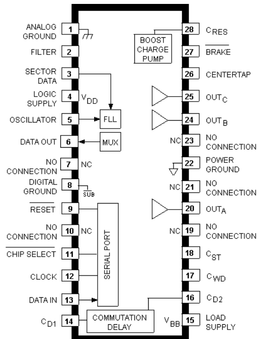
A8904SLP (TSSOP)
