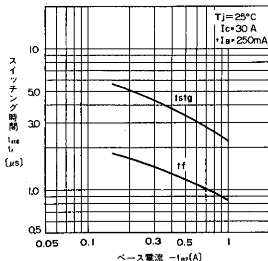
スウィッチング時間—ベース電流特性 Switching Time
