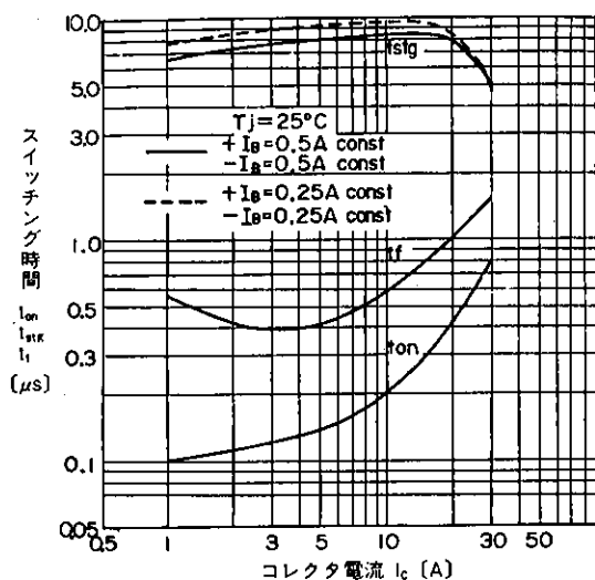
スウィッチング時間—コレクタ電流特性 Switching Time
