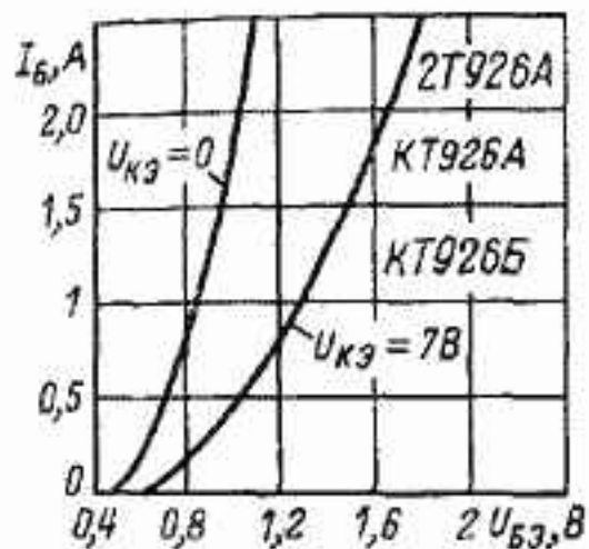
Входные характеристики.
