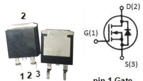
D 2 PAK
