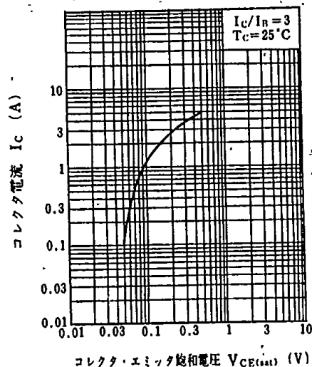
I_C - V_{CE(sat)}
