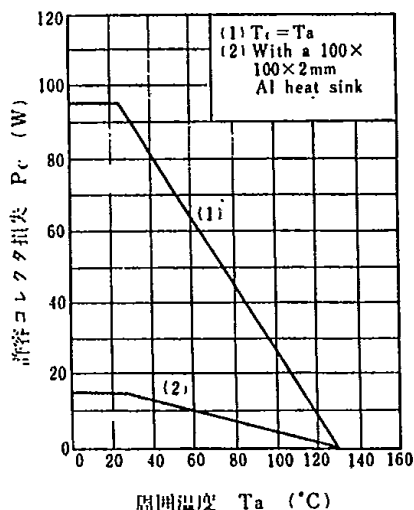
P_C - T_a
