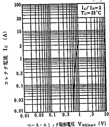
I_C - V_{BE(sat)}
