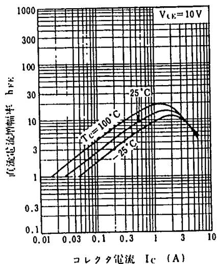
h_{FE} - I_C
