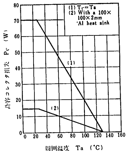
P_C - T_a
