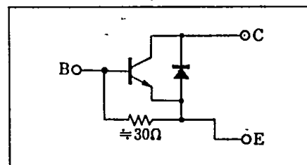
内部接続図 / Connection Diagram
