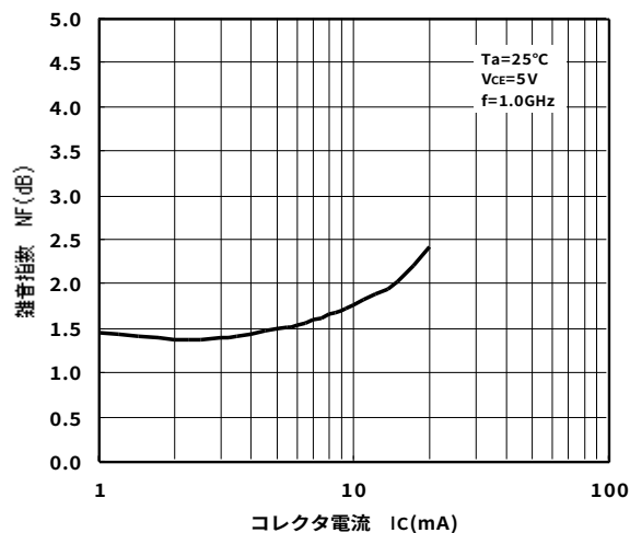
雑音指数-コレクタ電流特性
