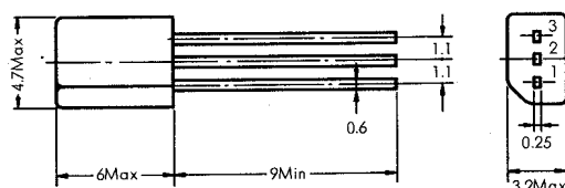
外形図 Plastic Mold
