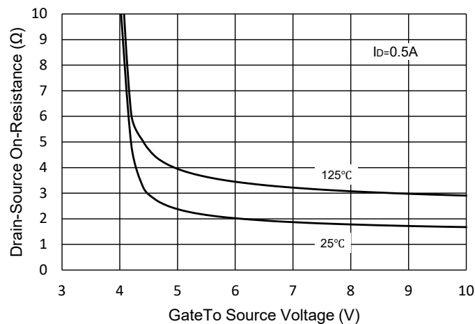
Fig.3 - R_{DS(on)} - V_{GS}
