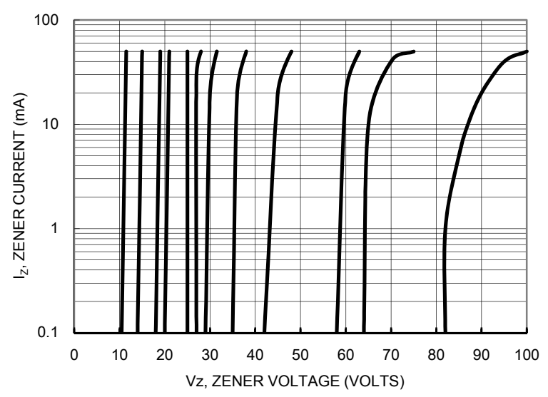
FIG. 7- Vz = 11 - 91 VOLTS
