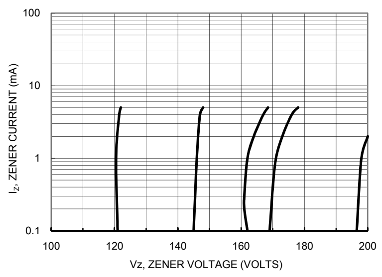
FIG. 8- Vz = 100 - 200 VOLTS
