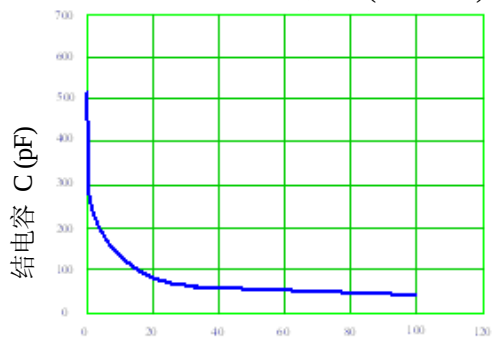
典型 C- V_R 关系曲线 (Per Diode)
