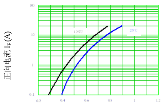
最大 I_F - V_F 关系曲线 (Per Diode)
