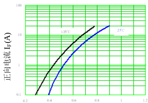
典型 I_F - V_F 关系曲线 (Per Diode)
