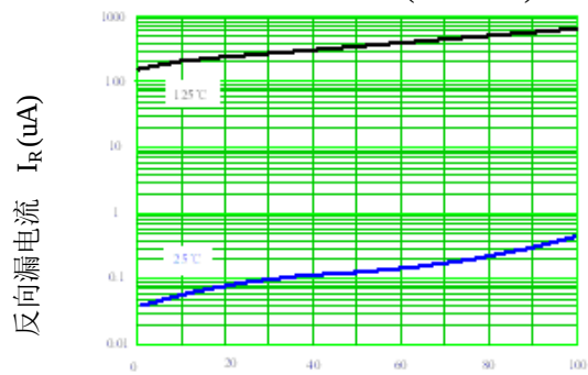
典型 I_R - V_R 关系特性 (Per Diode)
